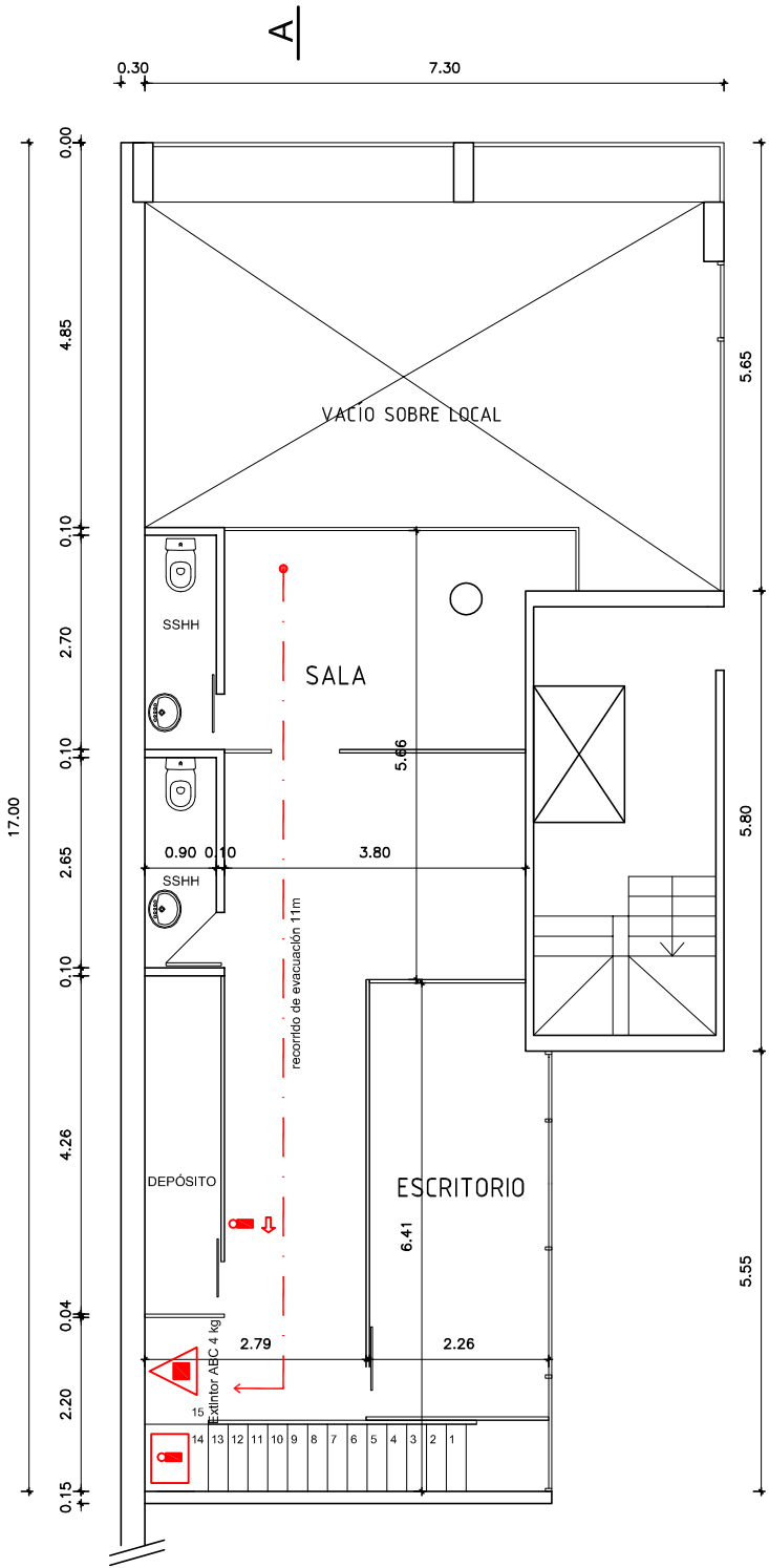
A PLANTA ALTA Sup. 56m 2 Esc. 1/100
